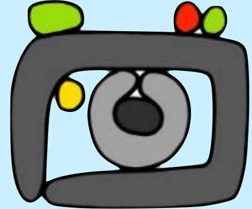
Fotoğraf Makinesi
